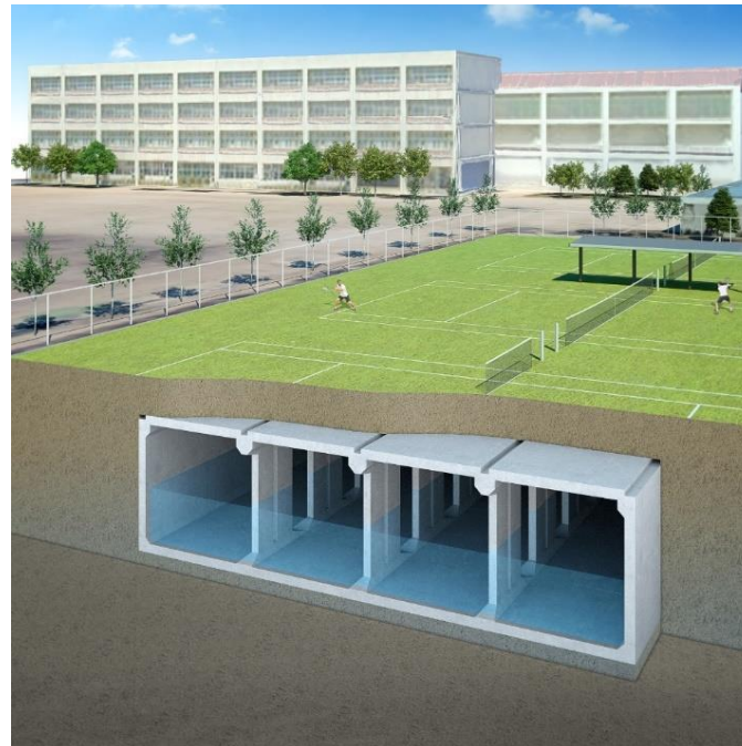
【大府北中学校調整池 イメージ図】
