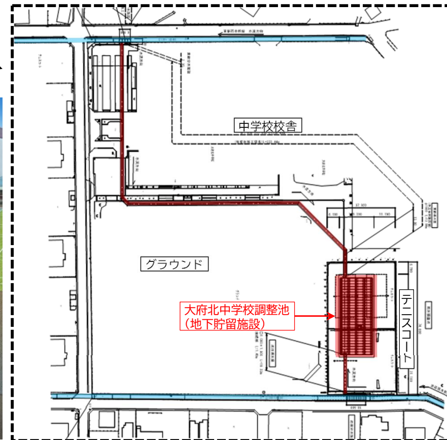
【平面図】
